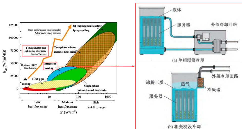
图1：单相浸没冷却和相变浸没冷却是两种主流的液冷方式
